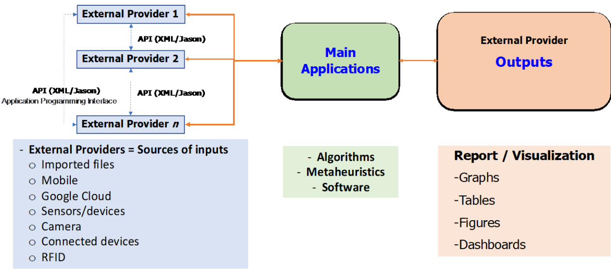
รูปที่ 1 สถาปัตยกรรมระบบ และการออกแบบโมดูลและส่วนประกอบที่จำเป็นในการประยุกต์ใช้ระบบ IoT ในรูปแบบการหาค่าเหมาะสมที่สุด (Optimization model)
